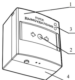
Рисунок 1 - Внешний вид УДП
