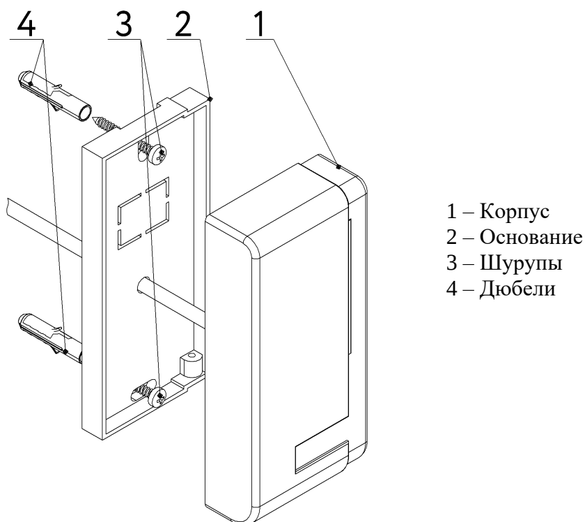
Рисунок 4 – Монтаж считывателя
