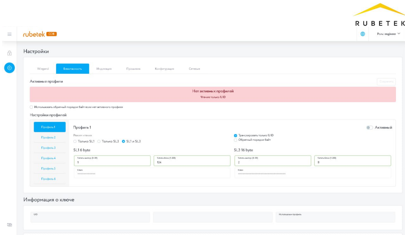
Рисунок 12 – Интерфейс страницы настроек безопасности
