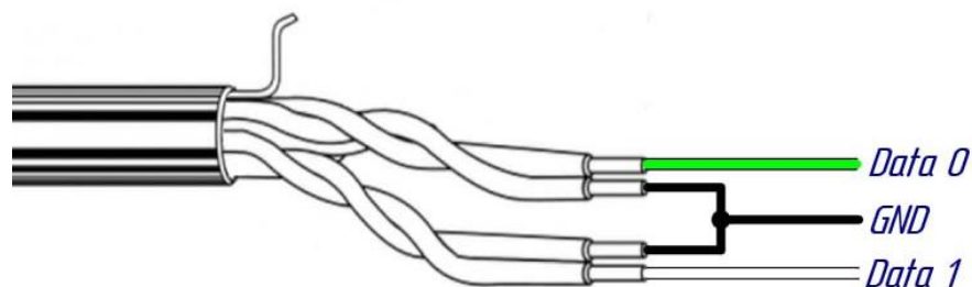
Рисунок 5 – Типовая схема подключения считывателя
