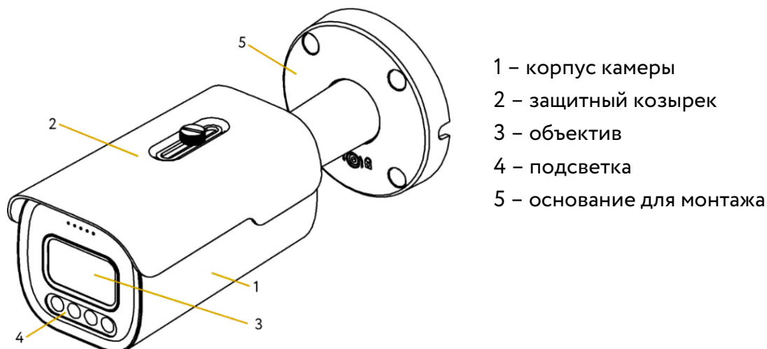
Рис. 1.1 – Внешний вид видеокамеры
