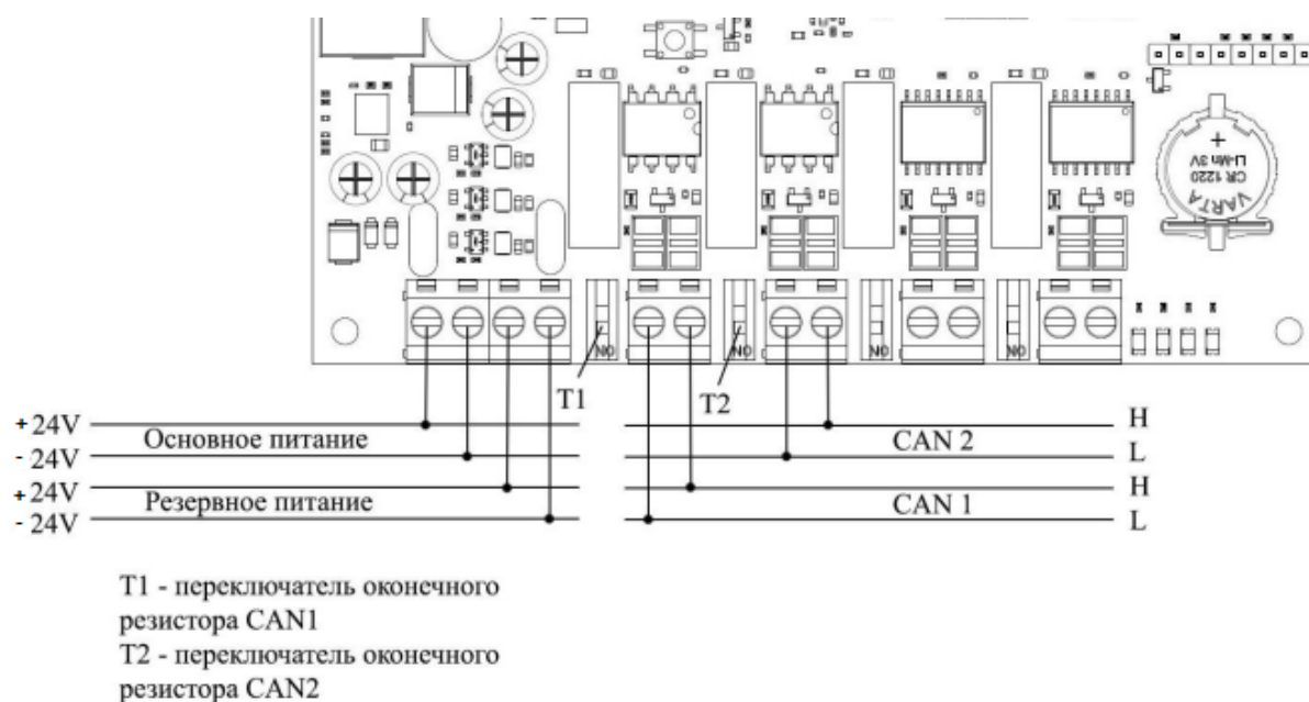
Рисунок 7 – Схема подключения интерфейса CAN и линии питания
