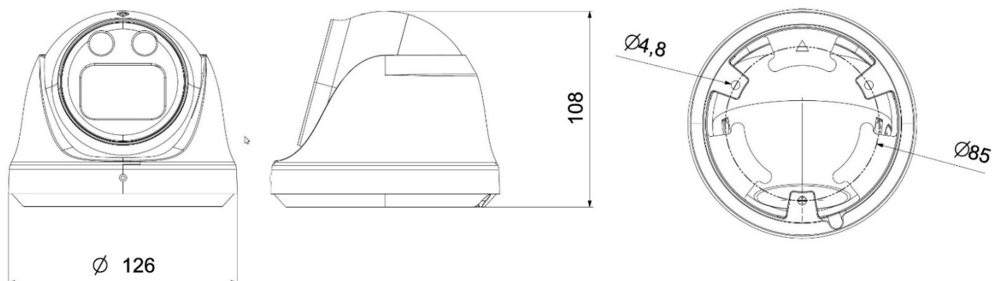
Рис. 2 – Габаритные размеры видеокамеры
